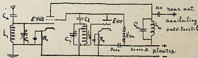
Fig. 2. Voorzetapparaat met wisselstroomlampen. Twee afstemmingen. Golf lengten vanaf 10 m.
